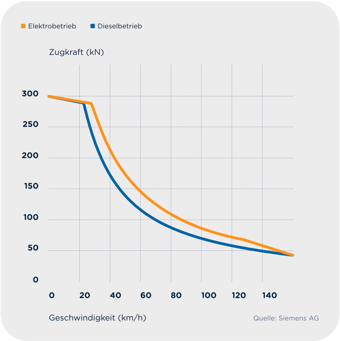
Zugkraft Diagramm Vectron Dual Mode
