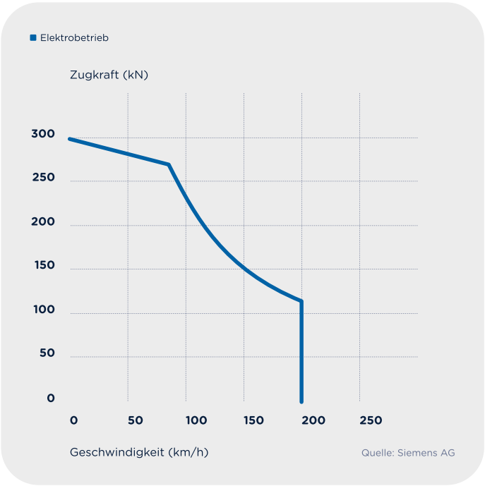
Zugkraft Diagramm Vectron AC
