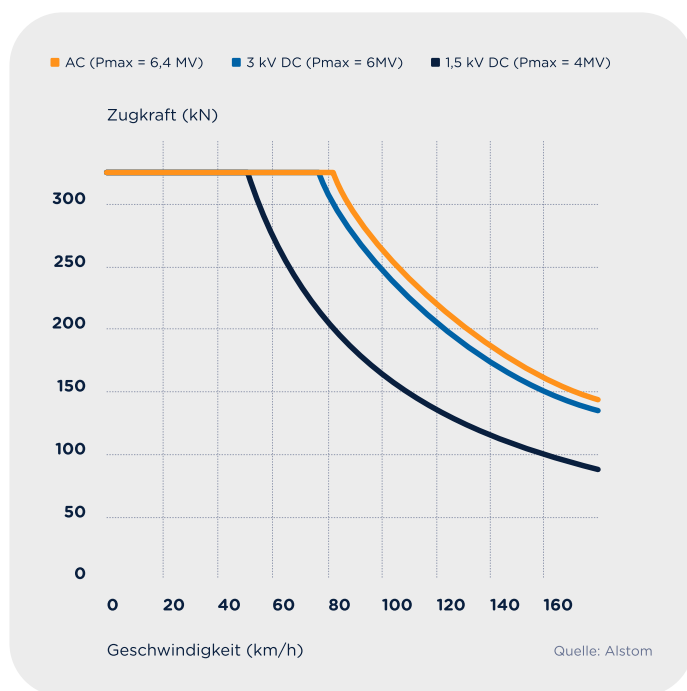
Zugkraft Diagramm Traxx 3 MS
