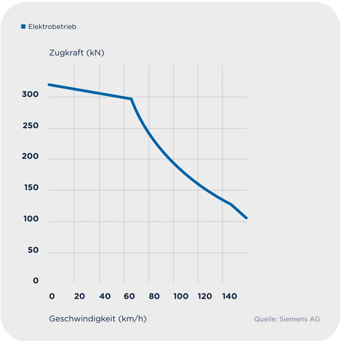
Zugkraft Diagramm Smartron
