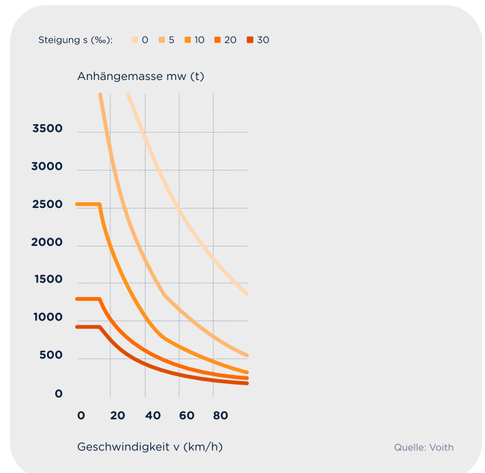
Anhängemasse Diagramm Gravita 15L
