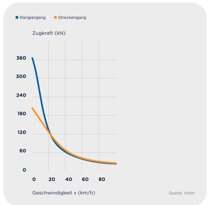
Zugkraft Diagramm Gravita 10
