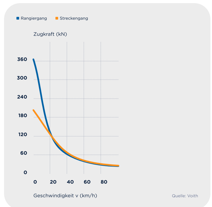
Zugkraft Diagramm Gravita 10
