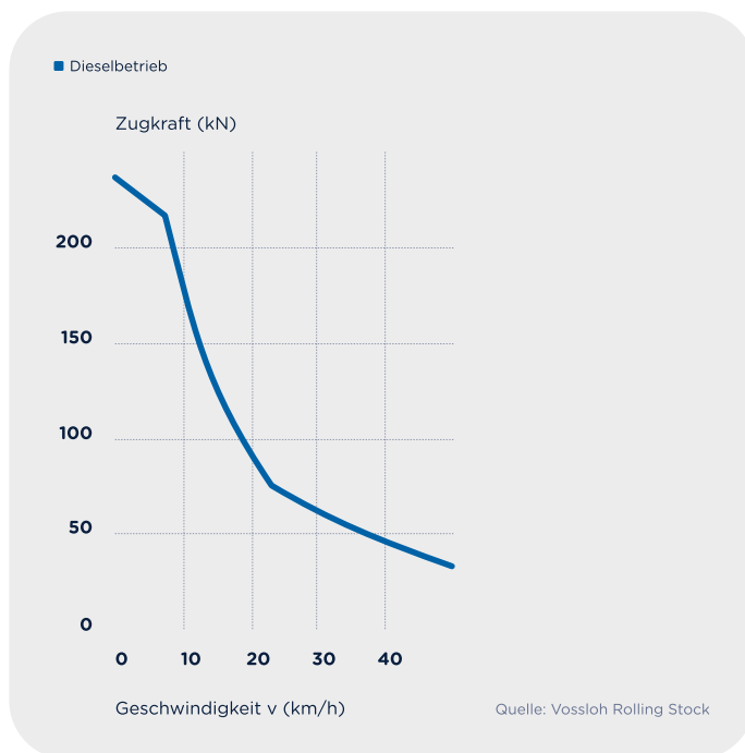
Zugkraft Diagramm G 800
