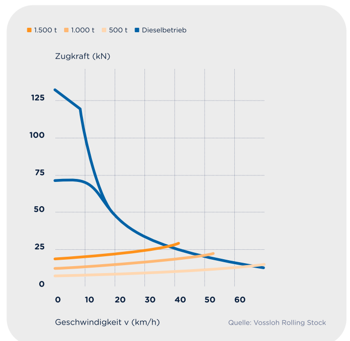
Zugkraft Diagramm G 322
