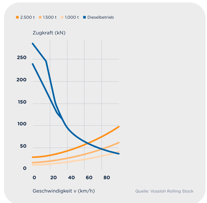
Zugkraft Diagramm G 1206
