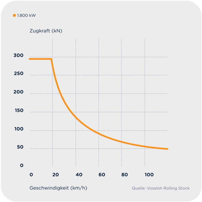
Zugkraft Diagramm DE 18
